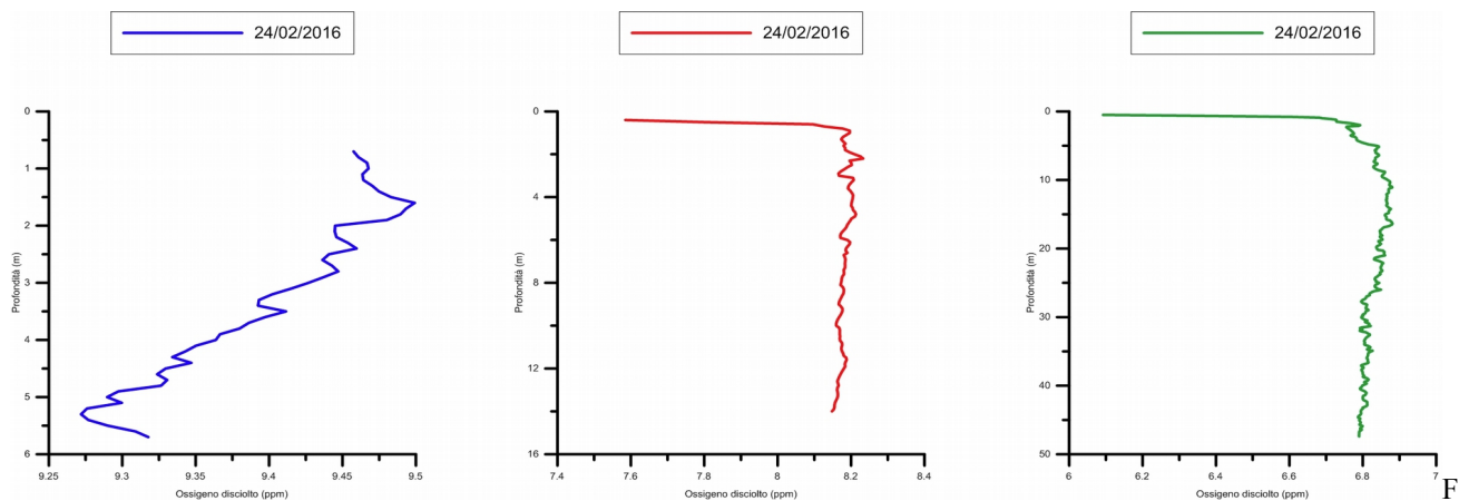
ig. 8 Andamento dell'Ossigeno disciolto nelle Stazioni ST03PT, ST02PT, ST01PT durante la campagna FPOA_15
