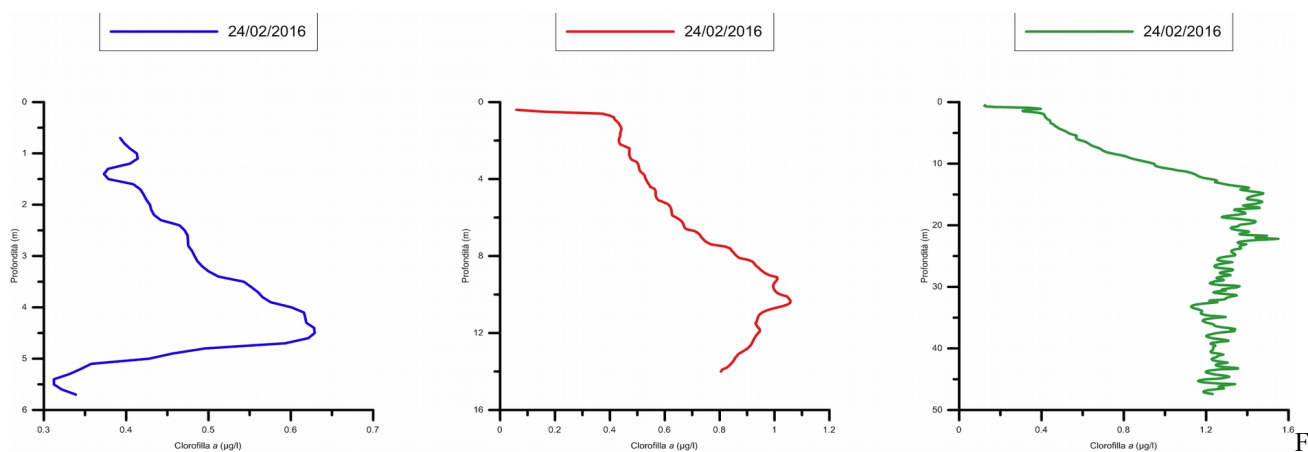
ig. 10 Andamento della clorofilla a nelle Stazioni ST03PT, ST02PT, ST01PT durante la campagna FPOA_15
