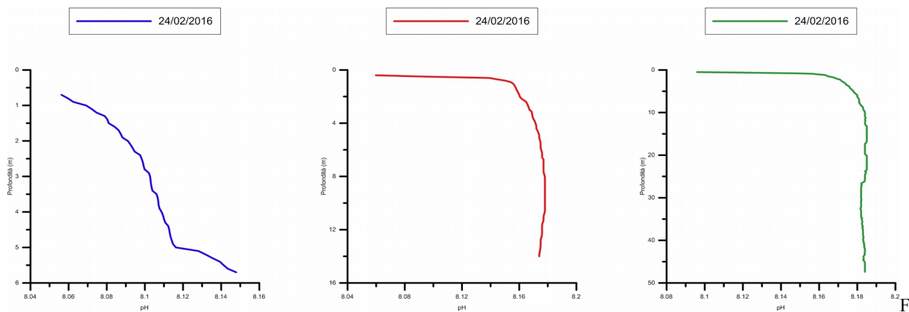
ig. 9 Andamento del pH nelle Stazioni ST03PT, ST02PT, ST01PT durante la campagna FPOA_15
