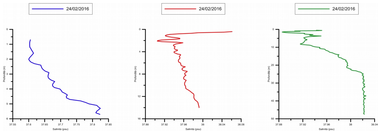
Fig. 6 Andamento della Salinità nelle Stazioni ST03PT, ST02PT, ST01PT durante la campagna FPOA_15
