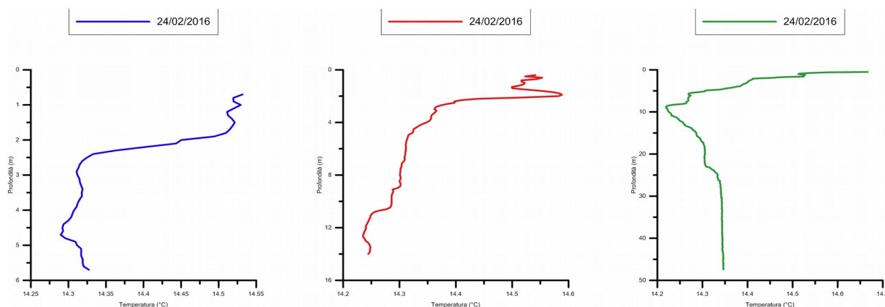
Fig. 4 Andamento della Temperatura nelle Stazioni ST03PT, ST02PT, ST01PT durante la campagna FPOA_15
