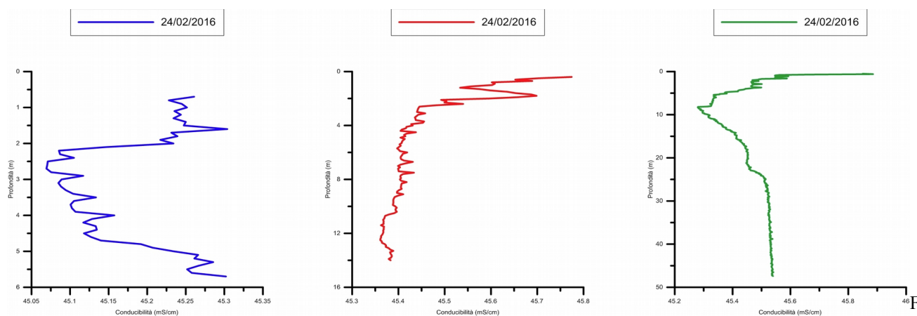
ig. 5 Andamento della Conducibilità nelle Stazioni ST03PT, ST02PT, ST01PT durante la campagna FPOA_15
